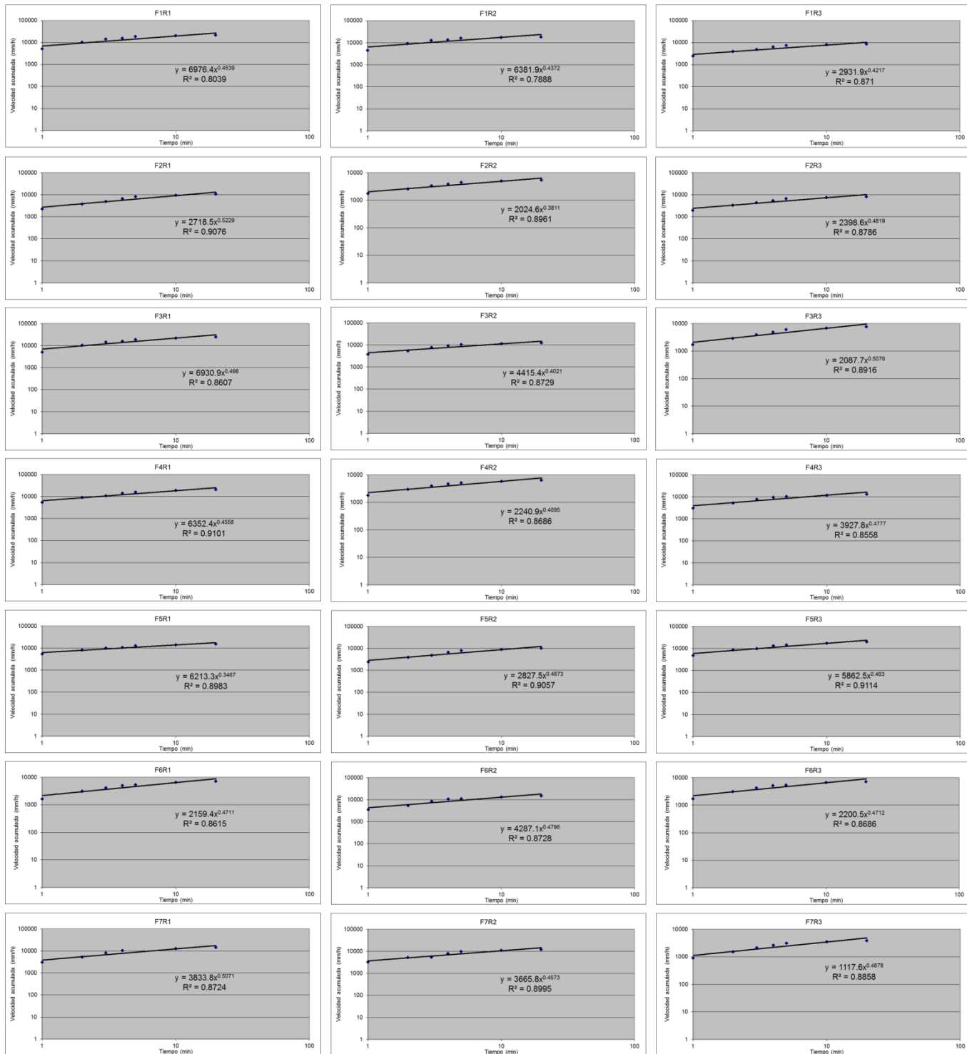
Figura 16. Velocidad de infiltración acumulada en siete fincas bajo cobertura de plantación pura de Pinus caribaea .
