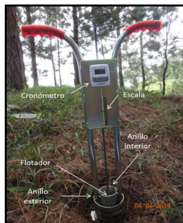
Figura 14. Infiltrómetro de doble anillo Turf-Tec. Fuente: Elaborado a partir de foto propia.
