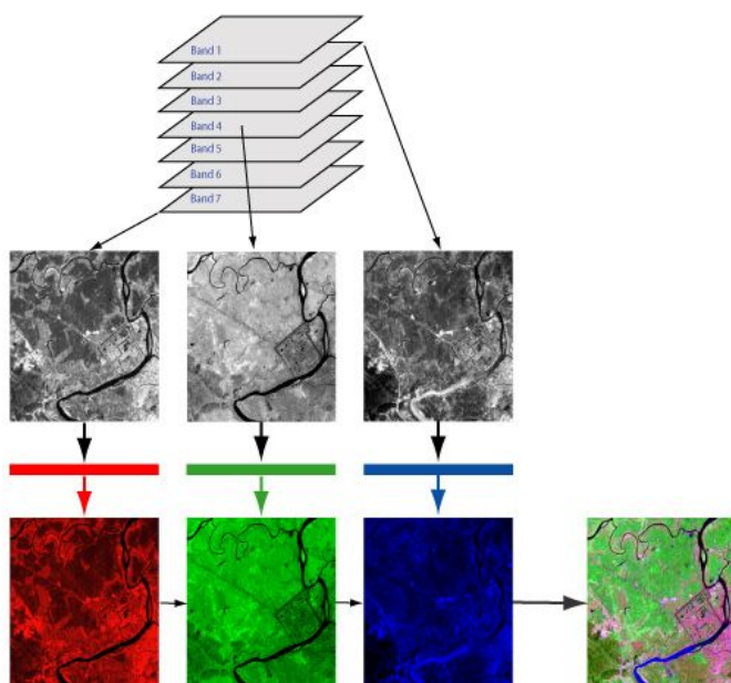
Figura 5.5: Combinación de datos de imágenes de tres canales de sensores para producir una imagen multispectral. Tales imágenes compuestas por colores ayudan en la visualización e interpretación de la cobertura de la tierra. Los niveles de brillo, que se muestran en tonos grises, representan los valores de cada canal.
