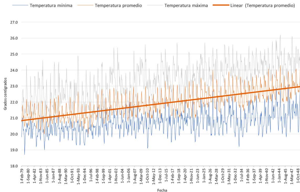
Figura 6. Temperatura del Cantón de Curridabat para el período histórico (1979-1999) y bajo escenarios de calentamiento global (RCP4.5) al año 2050 15
