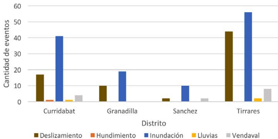
Figura 5. Tipos de desastres naturales de acuerdo con los distritos del cantón de Curridabat entre los años 1988-2018 (Fuente DesInventar y Municipalidad de Curridabat. 2015).
