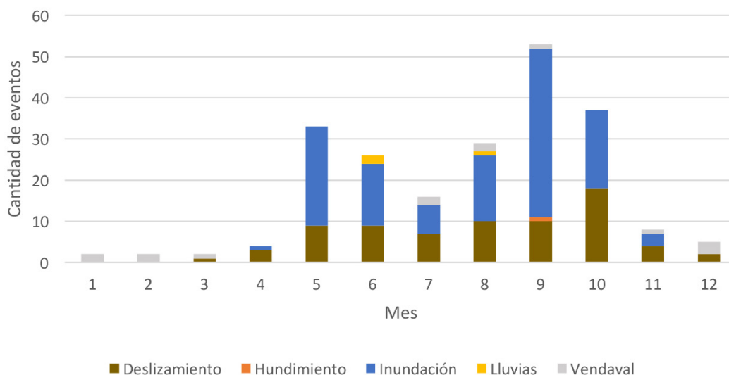
Figura 3. Tipo de evento y su incidencia de acuerdo con los meses del año entre 1988 - 2018, cantón de Curridabat (Fuente DesInventar y Municipalidad de Curridabat. 2015).
