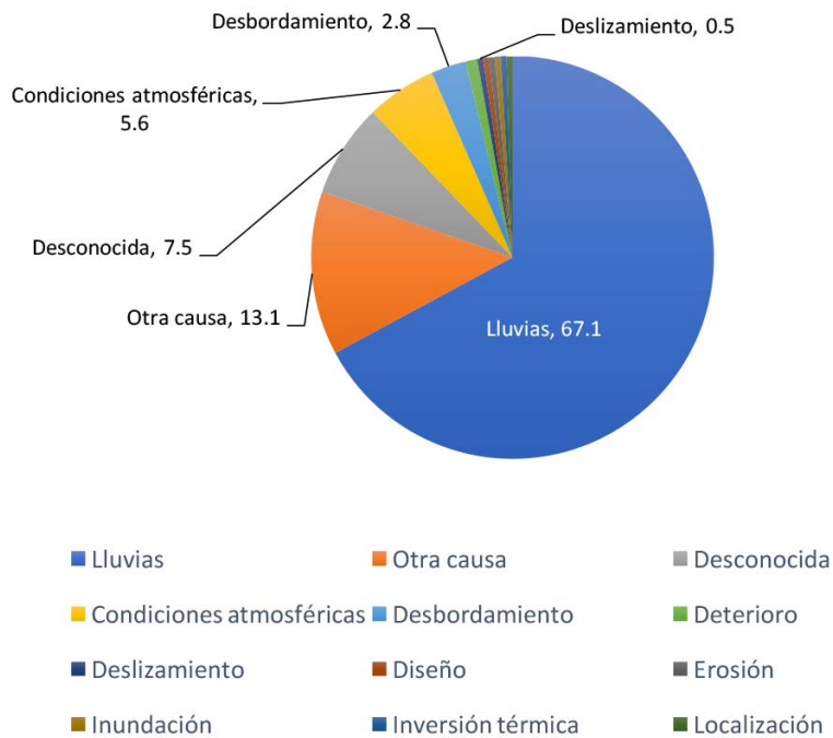
Figura 2. Origen de los eventos de desastres ocurridos en el cantón de Curridabat entre el año 1988-2018 (Fuente DesInventar y Municipalidad de Curridabat 2015)
