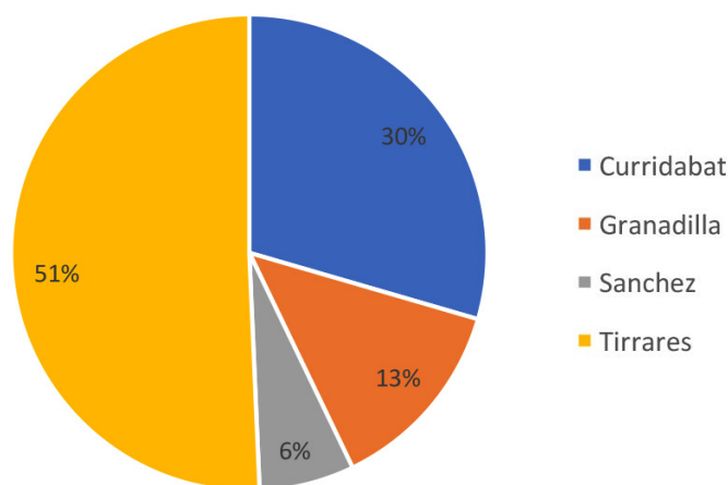
Figura 4. Proporción de desastres naturales según el distrito en el cantón de Curridabat en el período de 1988-2018 (Fuente DesInventar y Municipalidad de Curridabat. 2015).
