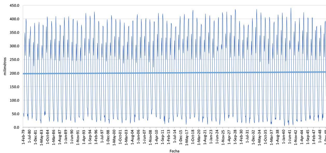
Figura 7. Precipitación acumulada del Cantón de Curridabat para el período histórico (1979-1999) y bajo escenarios de calentamiento global (RCP4.5) al año 2050 17 .
