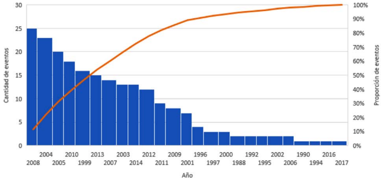
Figura 1. Eventos climáticos extremos del año 1988 al 2018 en el cantón de Curridabat (Fuente: DesInventar y Municipalidad de Curridabat. 2015).
