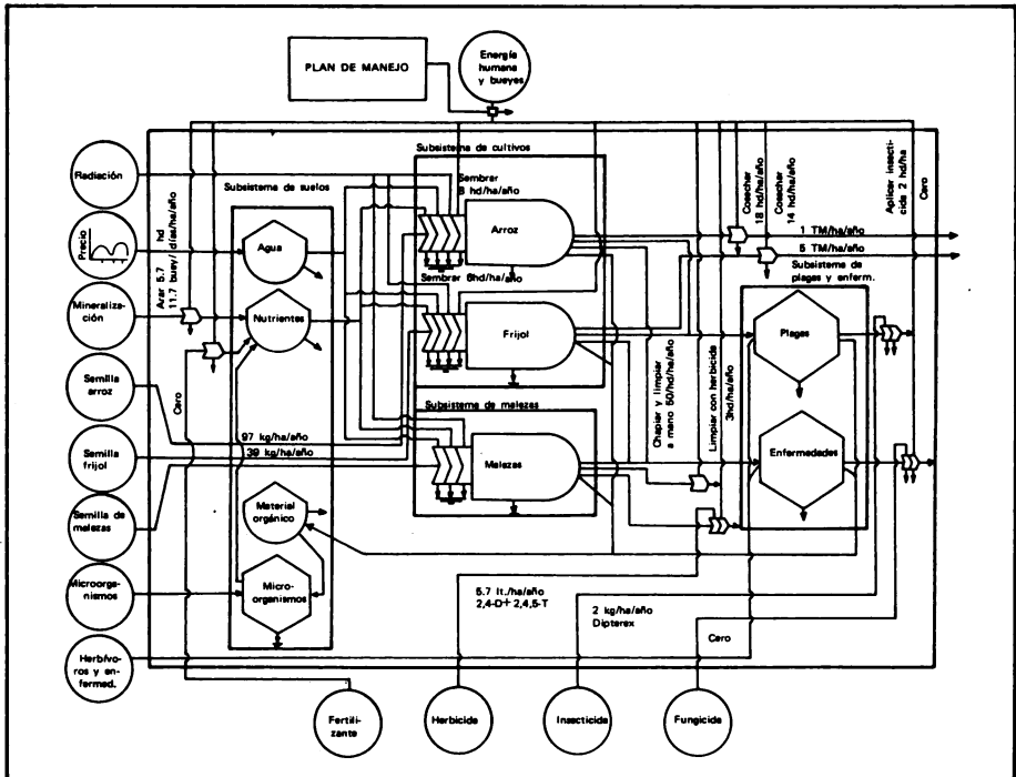
Figura 6.4 Diagrama semicualitativo de un agroecosistema con un subsistema de cultivos que incluye arroz y frijol en rotación. Las estimaciones de los diferentes flujos se dan en unidades/ha/año.
