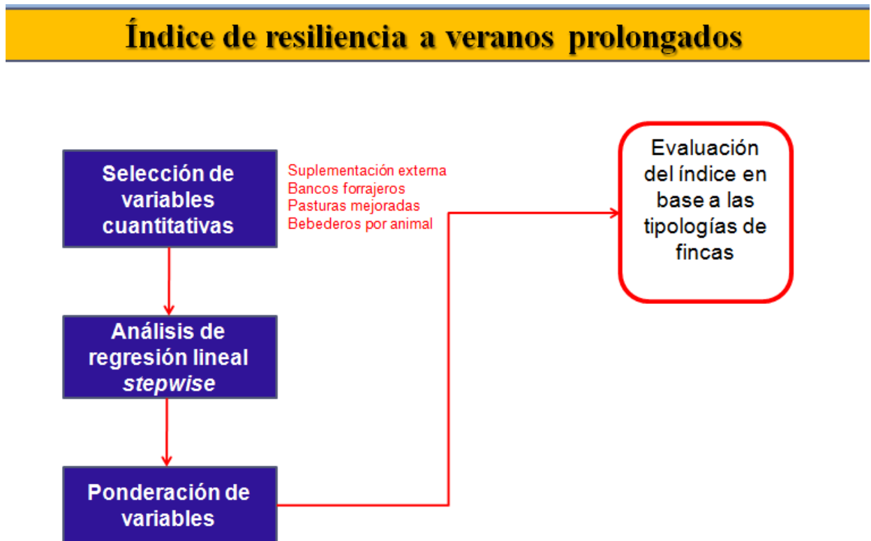
Figura 3. Pasos para la elaboración del índice de resiliencia a veranos prolongados.
