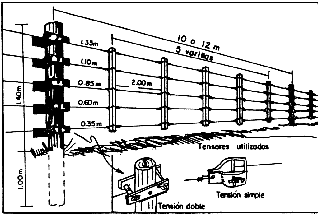
Figura 4. Cercas Eléctricas.
