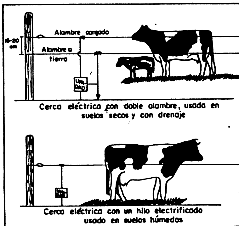
Figura 2. Formas de colocar una cerca eléctrica.
