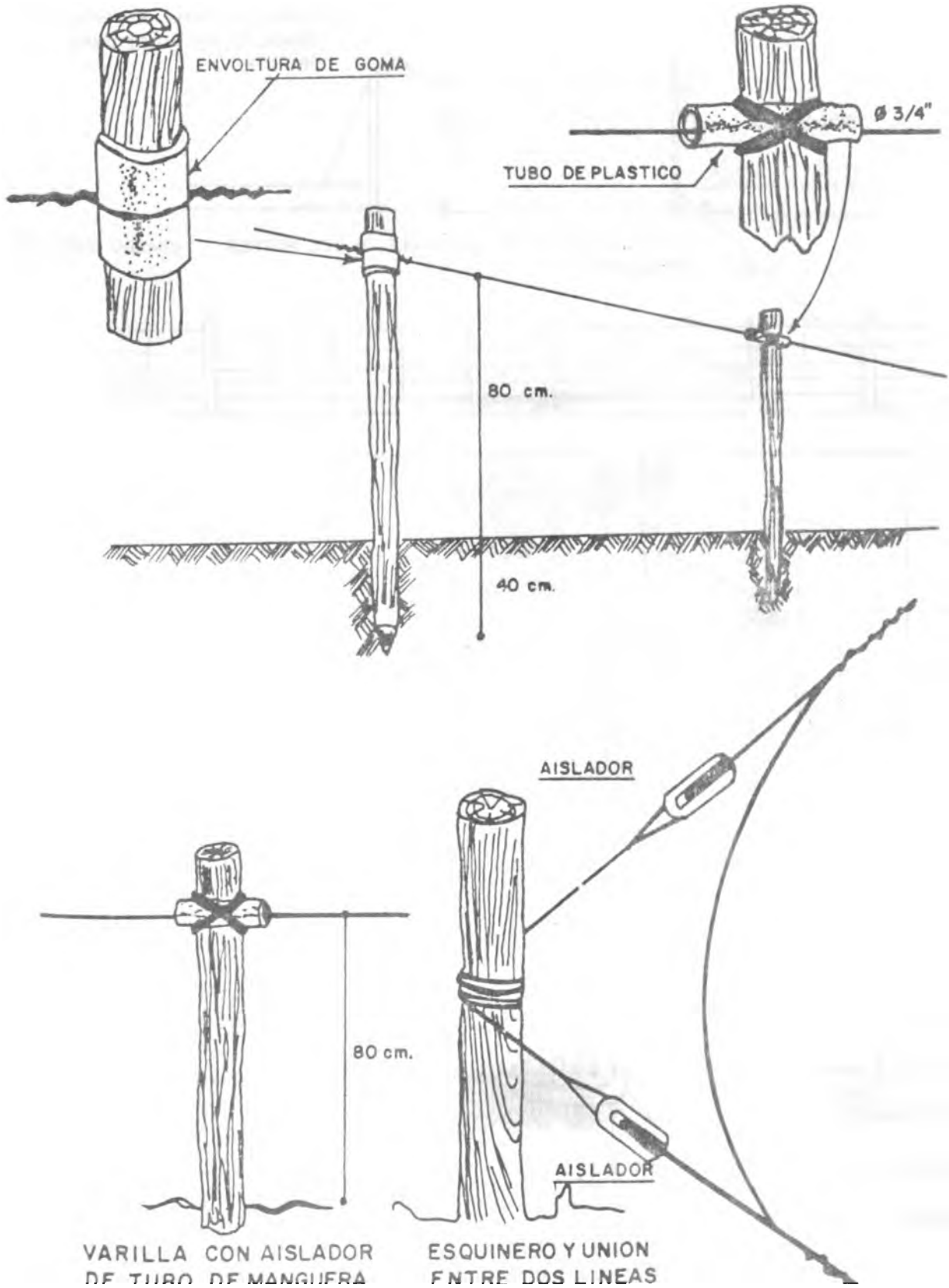
Figura 3. AISLADORES
