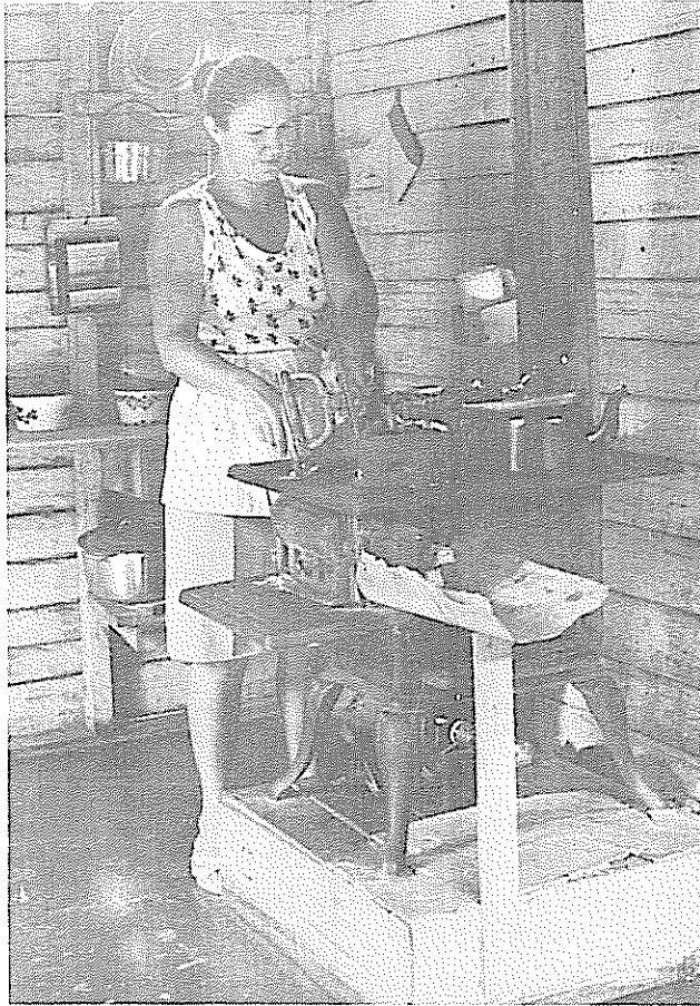
FOTO N° 7. La cocina de hierro, es la cocina de leña más usada en Costa Rica. La marca Perfection tiene diferentes modelos, y es fabricada en el país. (foto David Perry)
