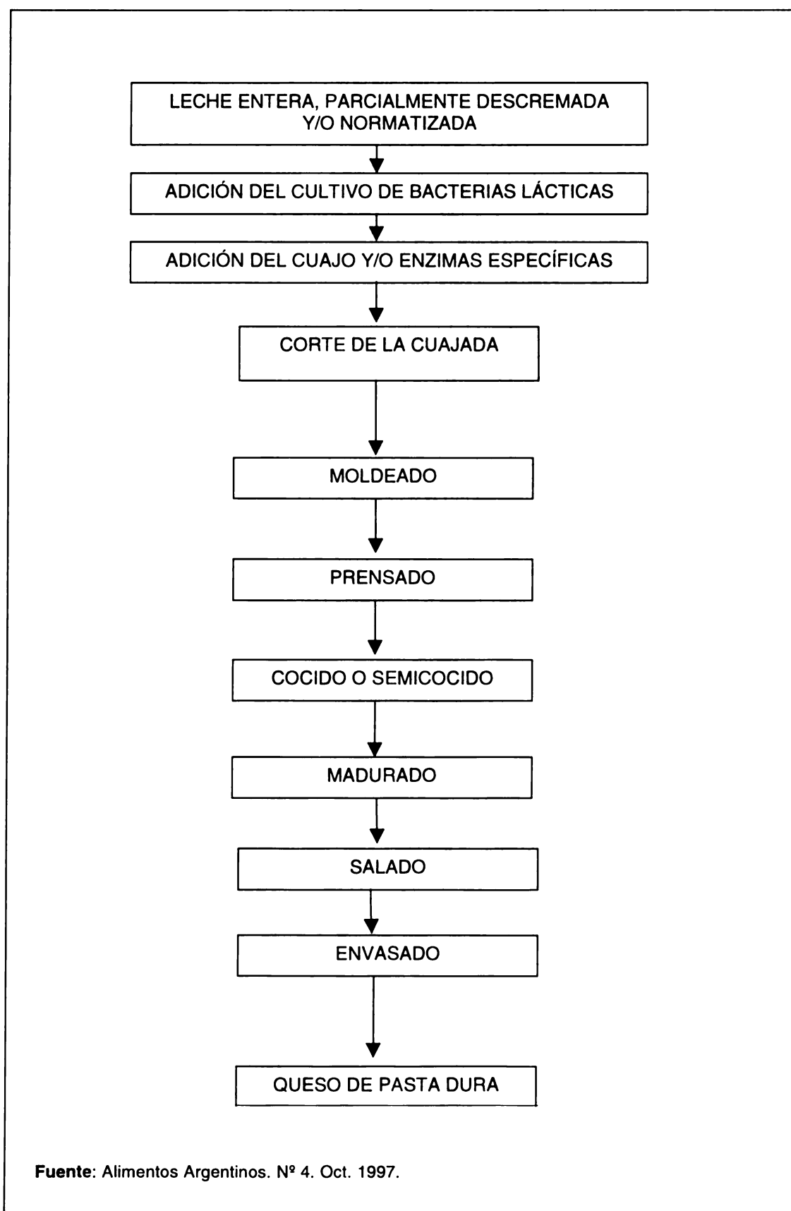
Figura 9. Producción de queso de pasta dura: cadena técnica
