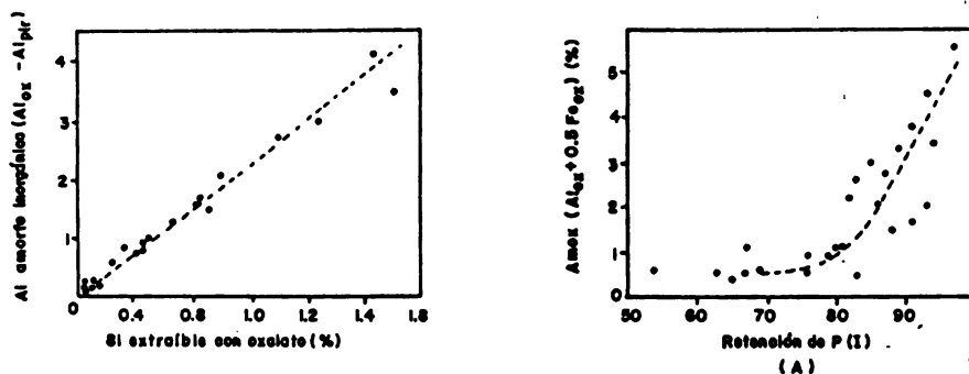
Fig. 1. Relación entre Si_{ox} y Al_{ox}-Al_{pir} en muestras de todos los suelos en la cronosecuencia.
