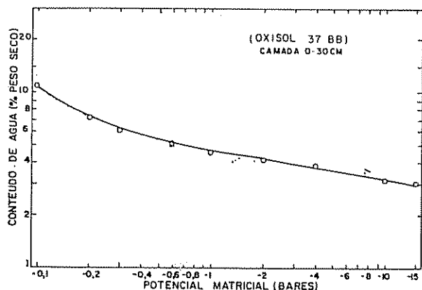
Fig. 1.—Curva de retenção de água do solo da área experimental
