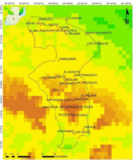
Índice de aridez para el municipio de San Miguel Chicaj (Escenario RCP 2.6 2080)
