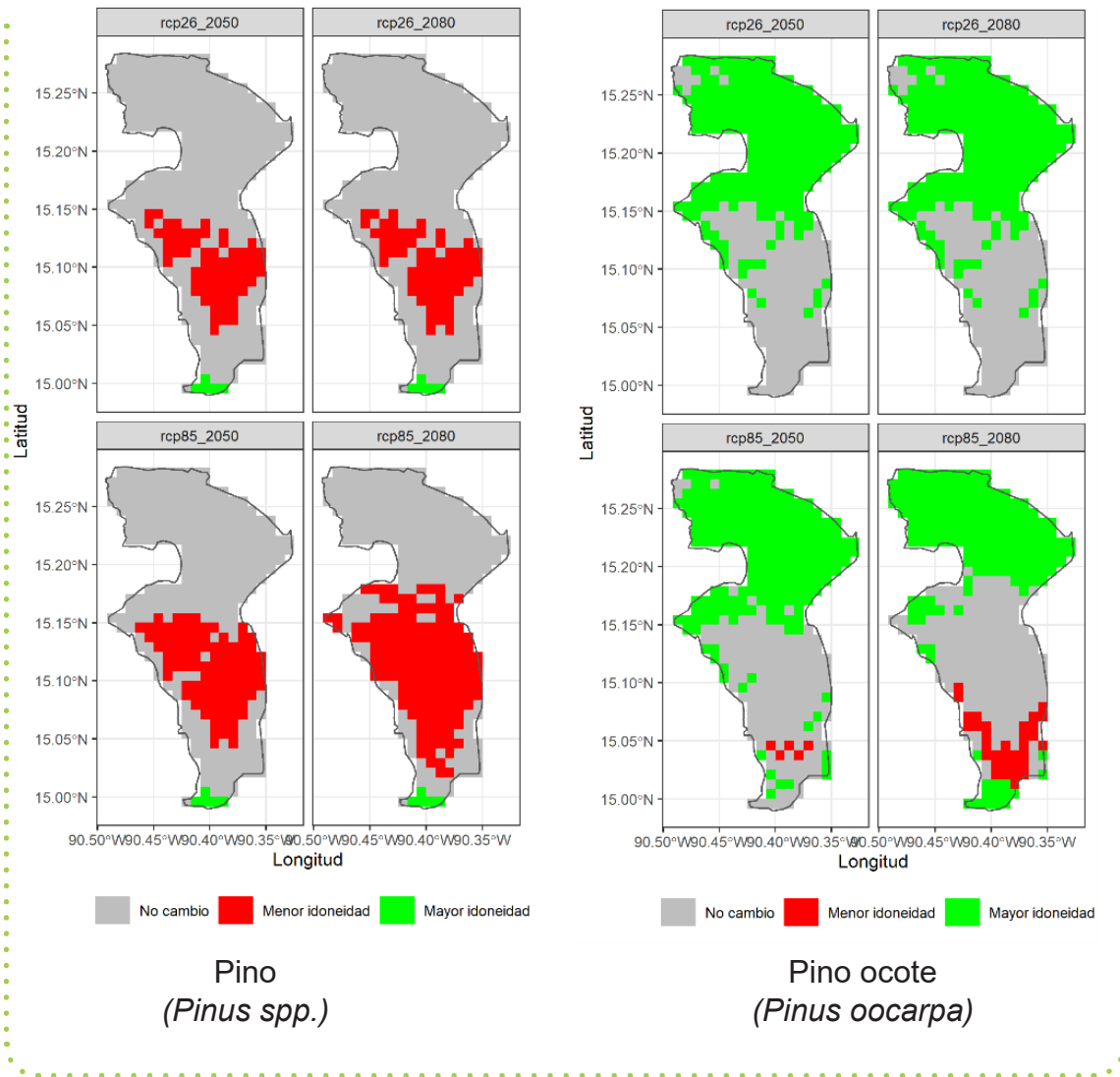
Figura 45. Cambios en la idoneidad climática del pino ( Pinus spp. ) y el pino ocote ( Pinus oocarpa ) en el municipio de San Miguel Chicaj, Baja Verapaz, Guatemala (climatología actual)
