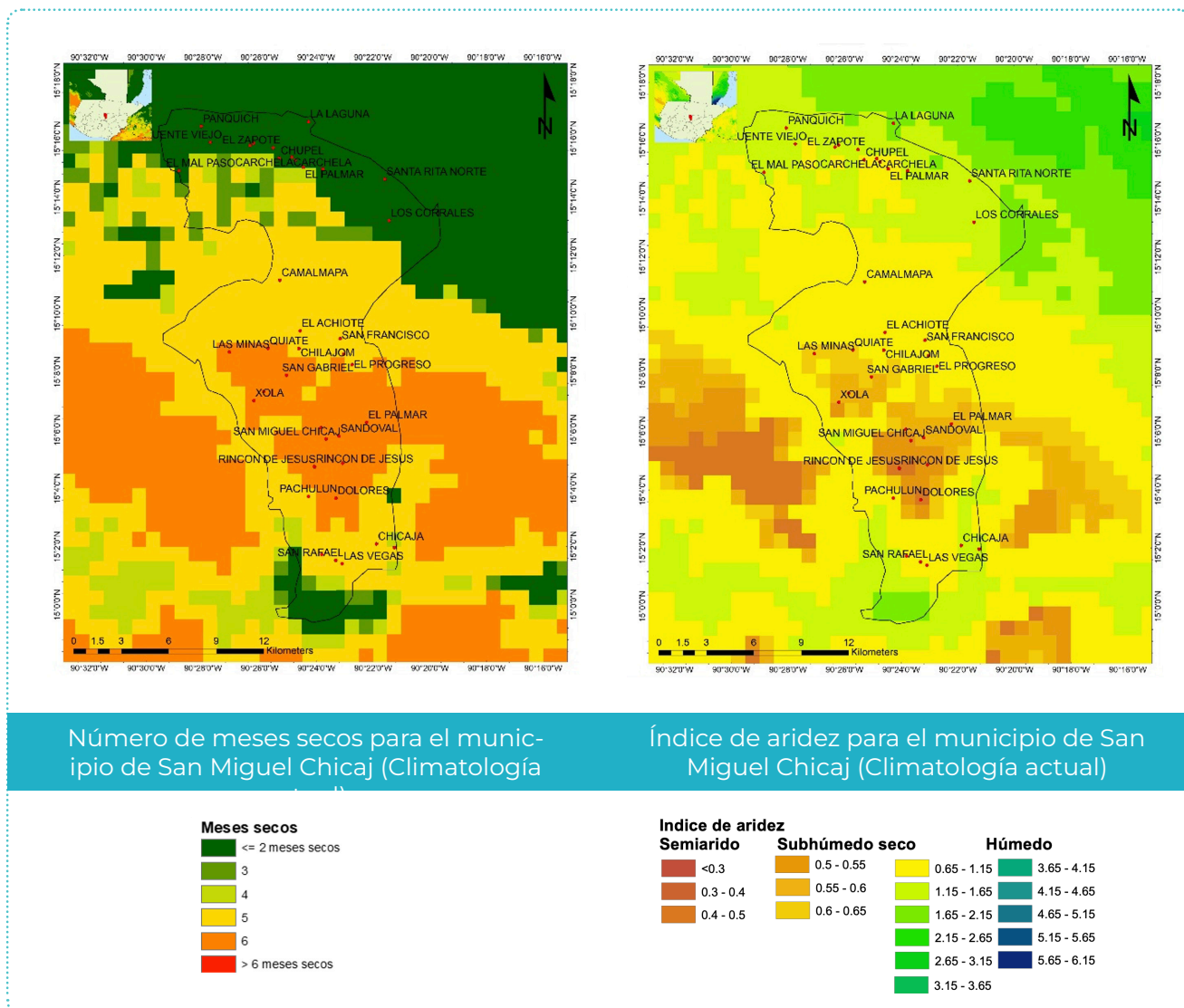
Figura 24. Número de meses secos, índice de aridez y evapotranspiración potencial en el municipio de San Miguel Chicaj (climatología 1960-1990)
