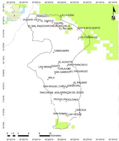
Índice de sensibilidad para el municipio de San Miguel Chicaj (Escenario RCP 8.5 2080)
