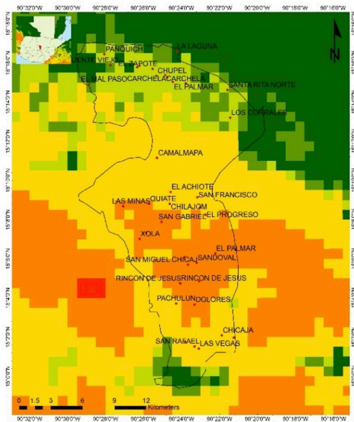
Número de meses secos para el municipio de San Miguel Chicaj (Escenario RCP 2.6 2050)
