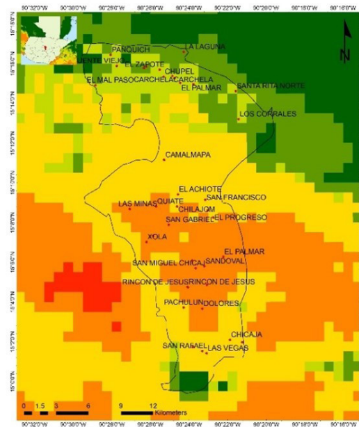
Número de meses secos para el municipio de San Miguel Chicaj (Escenario RCP 8.5 2050)
