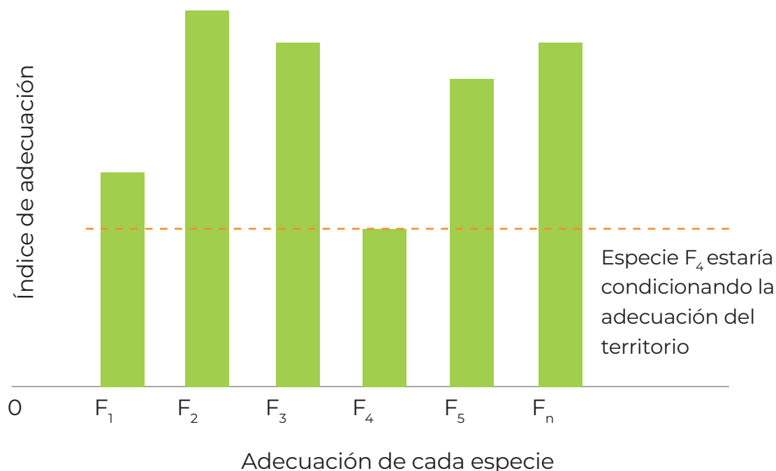
Figura 38. Adaptación de la ley de mínimo de Liebig al contexto de adecuación de espacial
