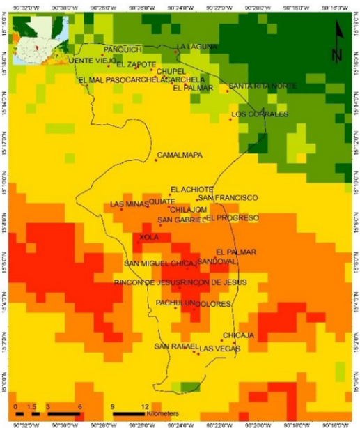
Número de meses secos para el municipio de San Miguel Chicaj (Escenario RCP 8.5 2080)
