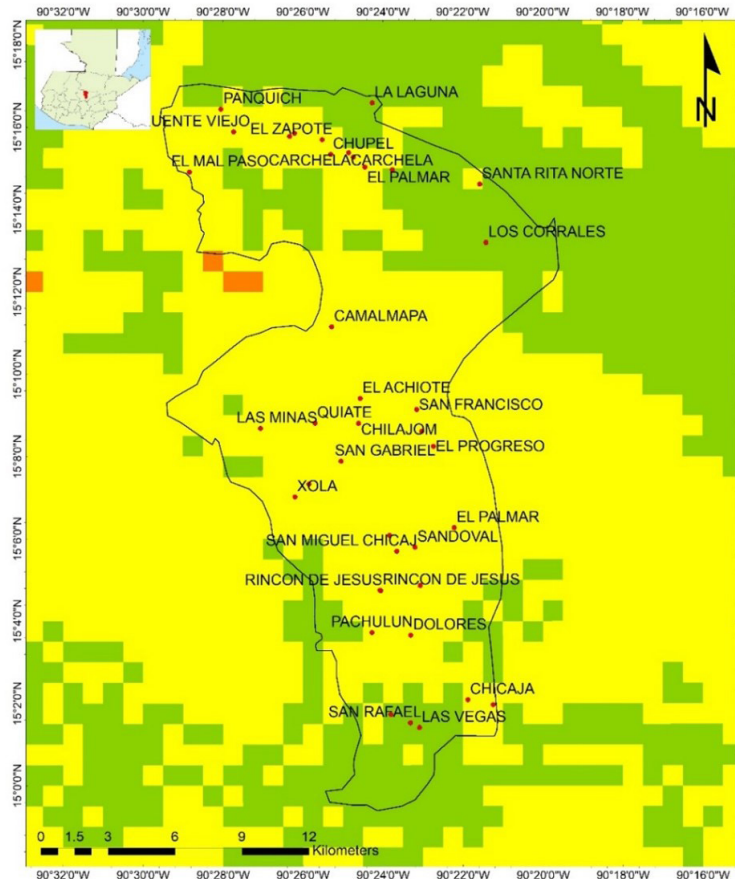
Mapa de riesgo climático RCP 2.6 2050
