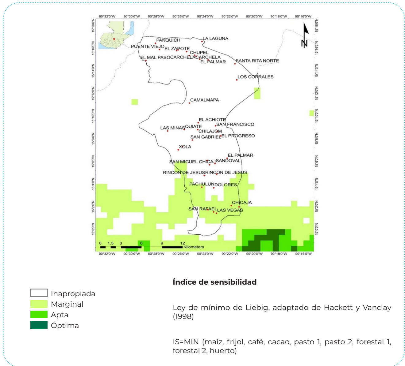
Figura 41. Índice de sensibilidad según climatología actual, con base en la adecuación de 9 especies a las condiciones climáticas del municipio de San Miguel Chicaj, Baja Verapaz, Guatemala
