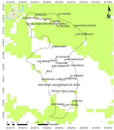
Índice de sensibilidad para el municipio de San Miguel Chicaj (Escenario RCP 2.6 2080)
