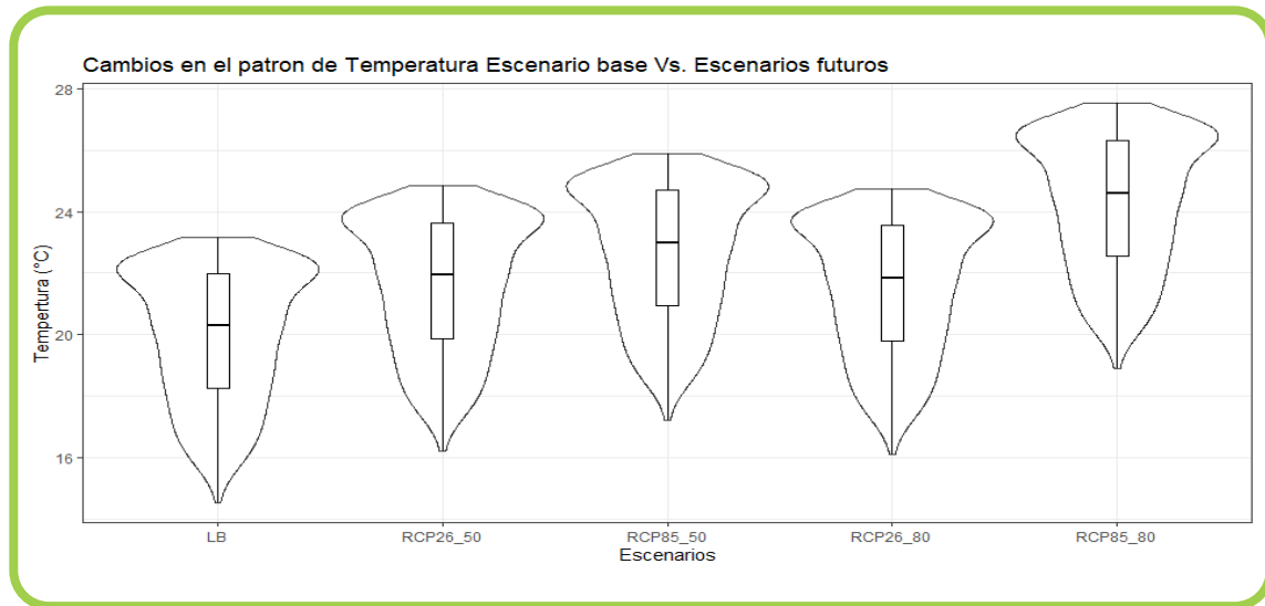
Figura 22. Comparación en la distribución de la temperatura promedio de la línea base y los escenarios futuros
