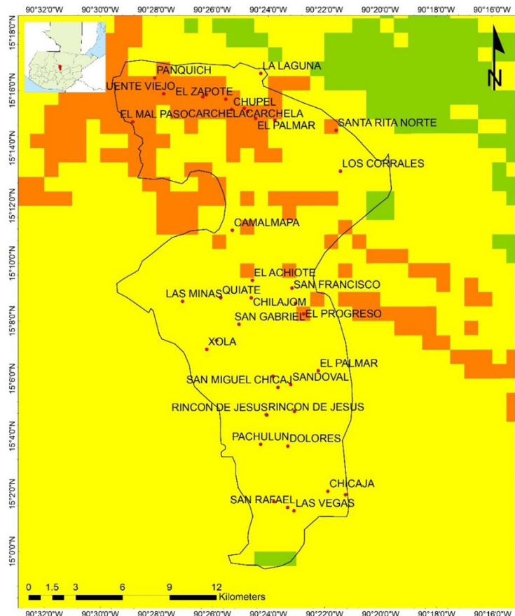
Mapa de riesgo climático RCP 8.5 2.80
