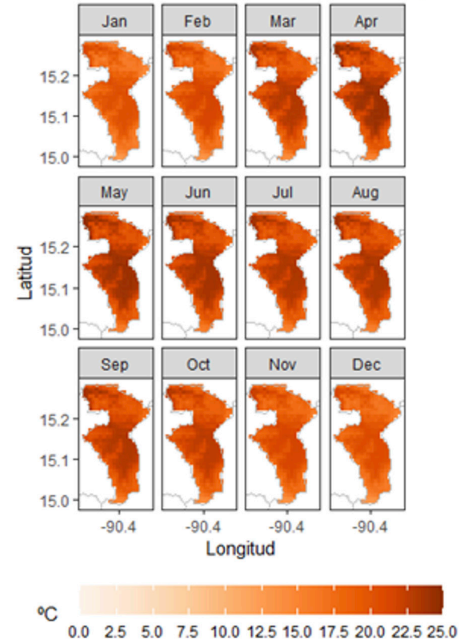
Temperatura media anual en San Miguel Chicaj (1960 - 1990)
