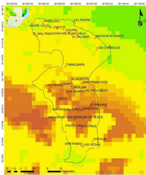
Índice de aridez para el municipio de San Miguel Chicaj (Escenario RCP 8.5 2050)
