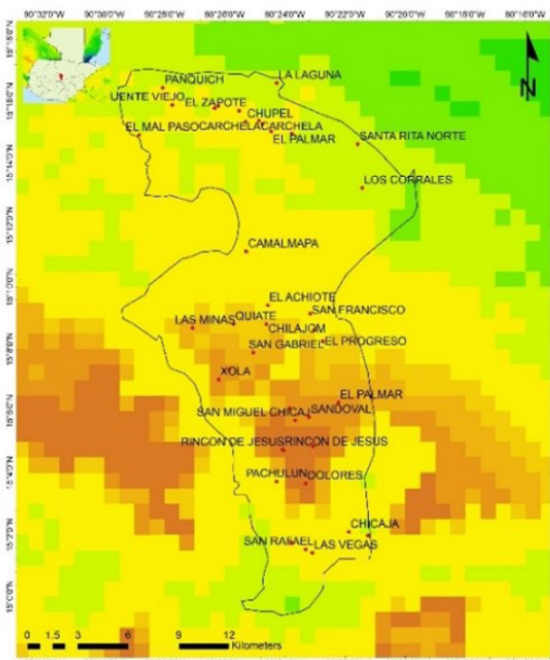
Índice de aridez para el municipio de San Miguel Chicaj (Escenario RCP 2.6 2050)
