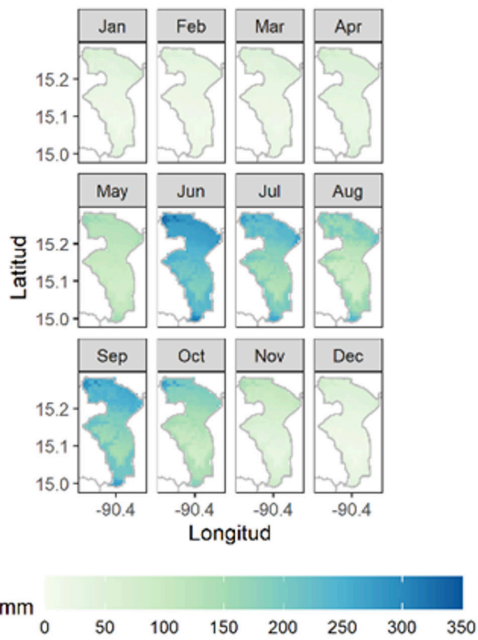
Precipitación mensual en San Miguel Chicaj (1960 - 1990)
