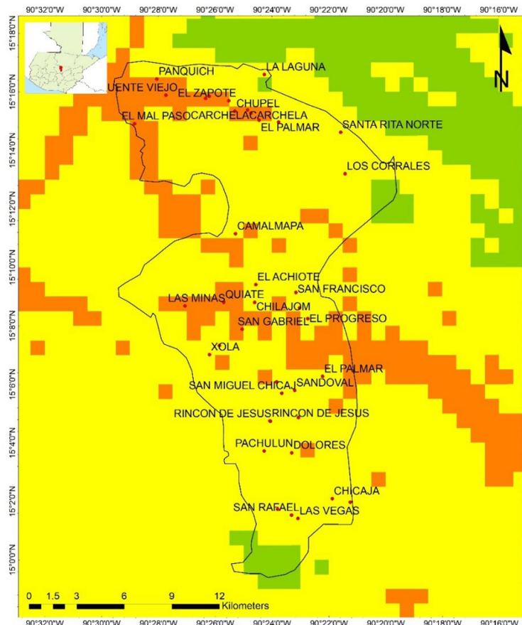
Mapa de riesgo climático RCP 8.5 2050
