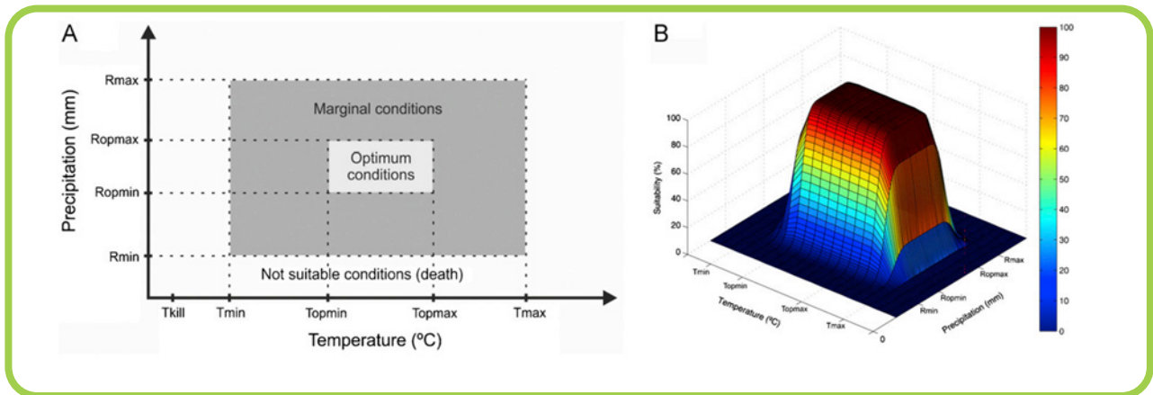
Figura 37. Representación en dos (A) y tres dimensiones (B) del modelo mecanístico usado en este análisis
