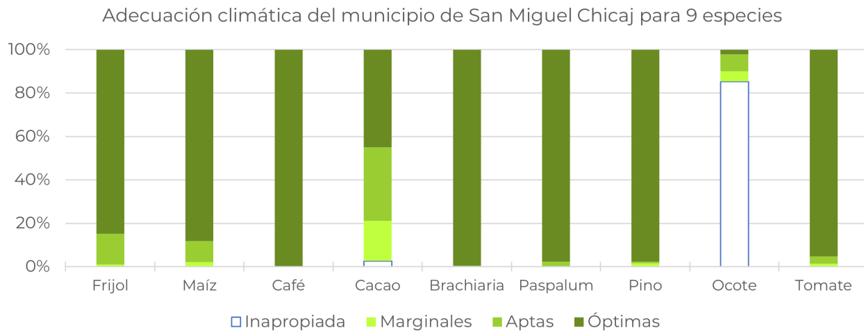
Figura 39. Adecuación climática de 9 especies en el municipio de San Miguel Chicaj, Baja Verapaz, Guatemala (climatología actual)
