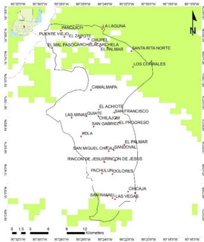
Índice de sensibilidad para el municipio de San Miguel Chicaj (Escenario RCP 8.5 2050)
