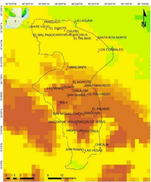
Índice de aridez para el municipio de San Miguel Chicaj (Escenario RCP 8.5 2080)
