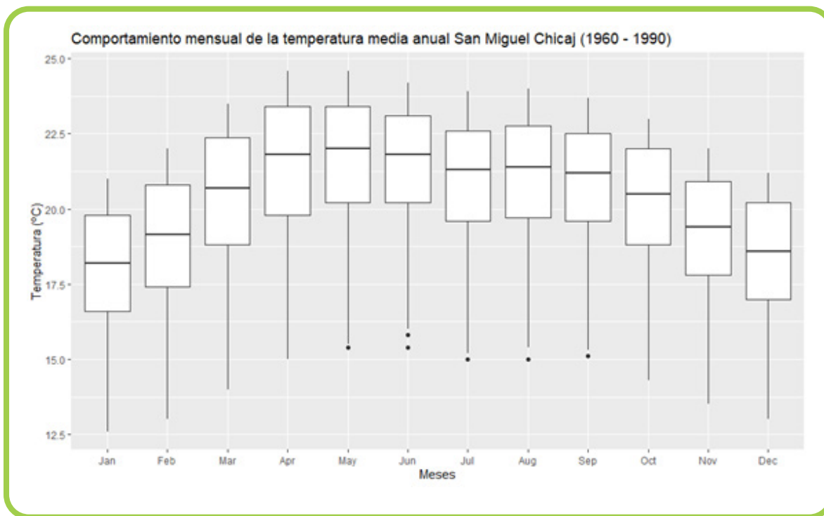
Figura 19. Variabilidad mensual de la temperatura promedio en San Miguel Chicaj, Baja Verapaz, Guatemala, según climatología 1960-1990
