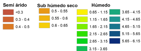
Figura 26. Cambios en el índice de aridez, entre la línea base y los escenarios futuros para San Miguel Chicaj, Baja Verapaz, Guatemala
