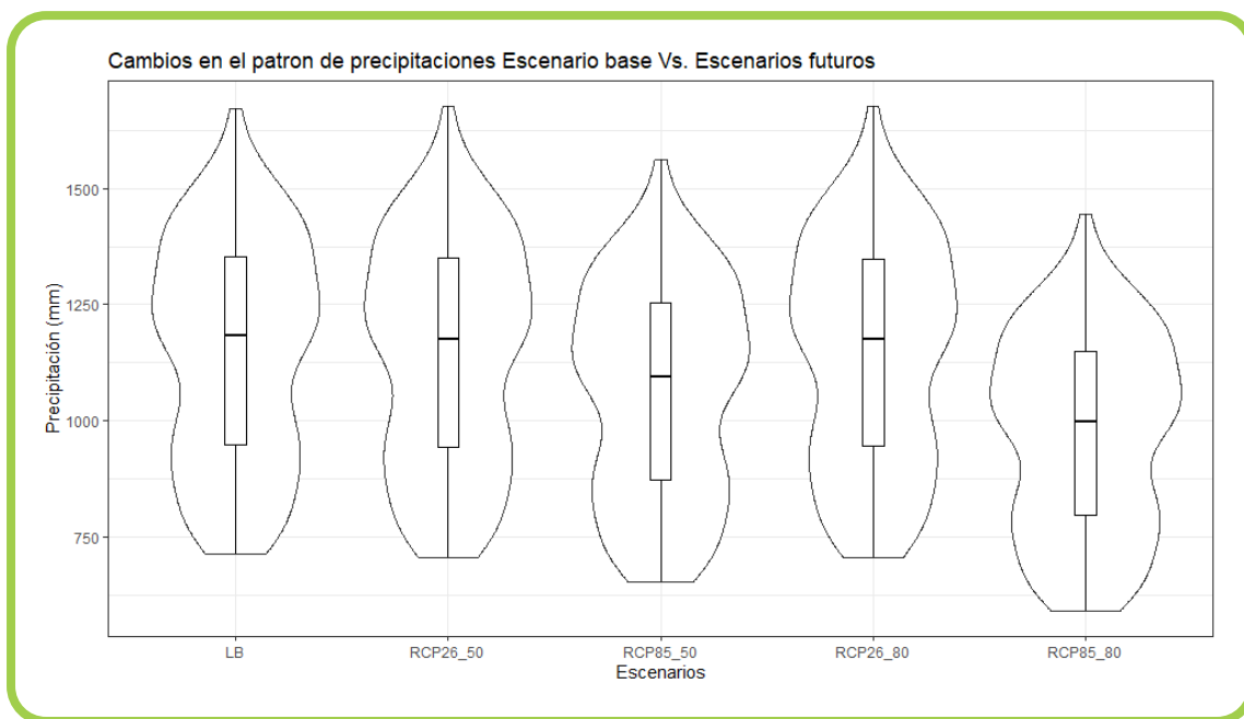
Figura 21. Comparación en la distribución de la precipitación total de la línea base y los escenarios futuros
