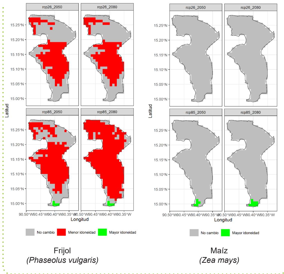
Figura 42. Cambios en la idoneidad climática del frijol ( Phaseolus vulgaris ) y el maíz ( Zea mays ) en el municipio de San Miguel Chicaj, Baja Verapaz, Guatemala (climatología actual)
