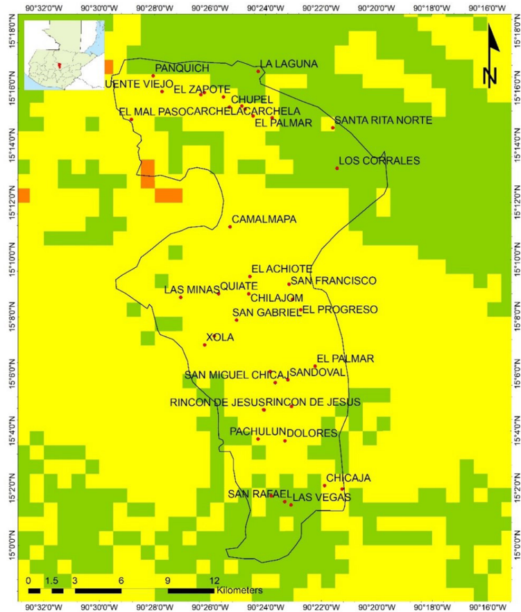
Mapa de riesgo climático RCP 2.6 2080
