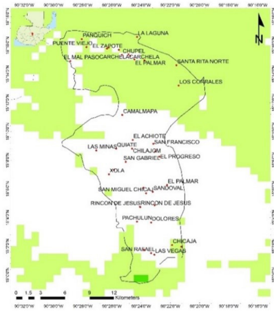
Índice de sensibilidad para el municipio de San Miguel Chicaj (Escenario RCP 2.6 2050)
