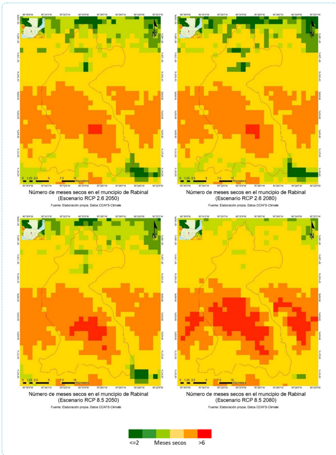
Figura 25. Número de meses secos según escenarios futuros para Rabinal, Baja Verapaz, Guatemala
