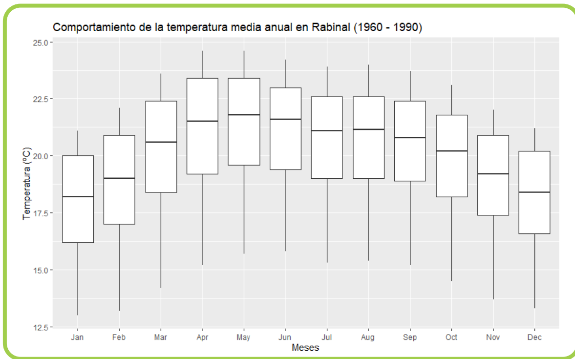
Figura 19. Variabilidad mensual de la temperatura promedio en Rabinal, Baja Verapaz, Guatemala, según climatología 1960-1990
