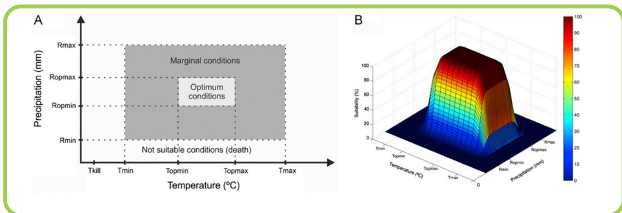
Figura 39. Representación en dos (A) y tres dimensiones (B) del modelo mecanístico usado en este análisis
