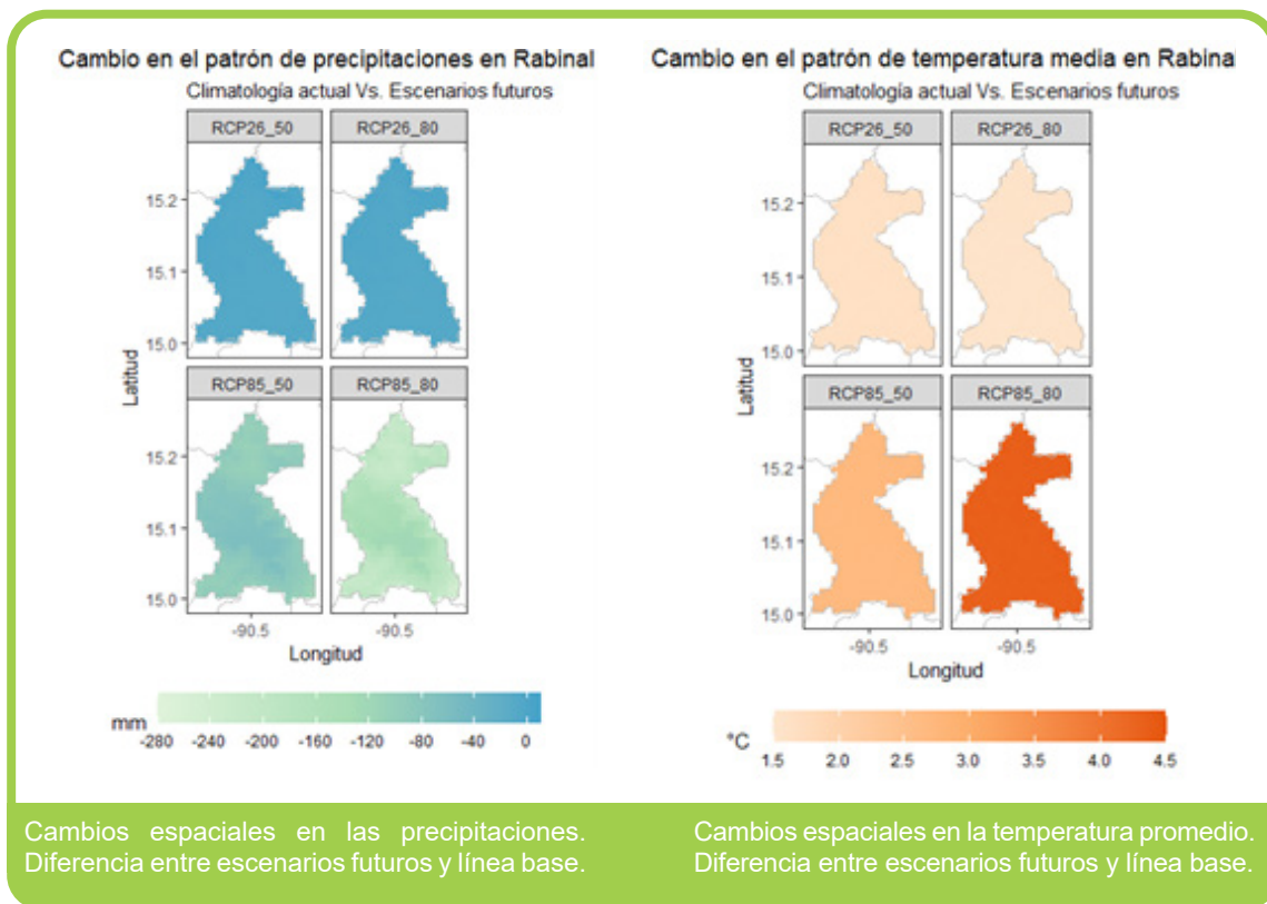
Figura 20. Cambios proyectados en las precipitaciones totales y la temperatura promedio en el municipio de Rabinal, Baja Verapaz, Guatemala, según RCP y horizonte temporal
