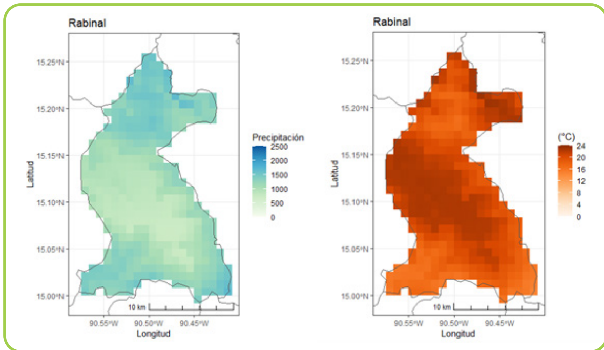
Figura 16. Mapa de distribución de la precipitación total y temperatura promedio en el municipio de Rabinal, Baja Verapaz, Guatemala, según climatología 1960-1990
