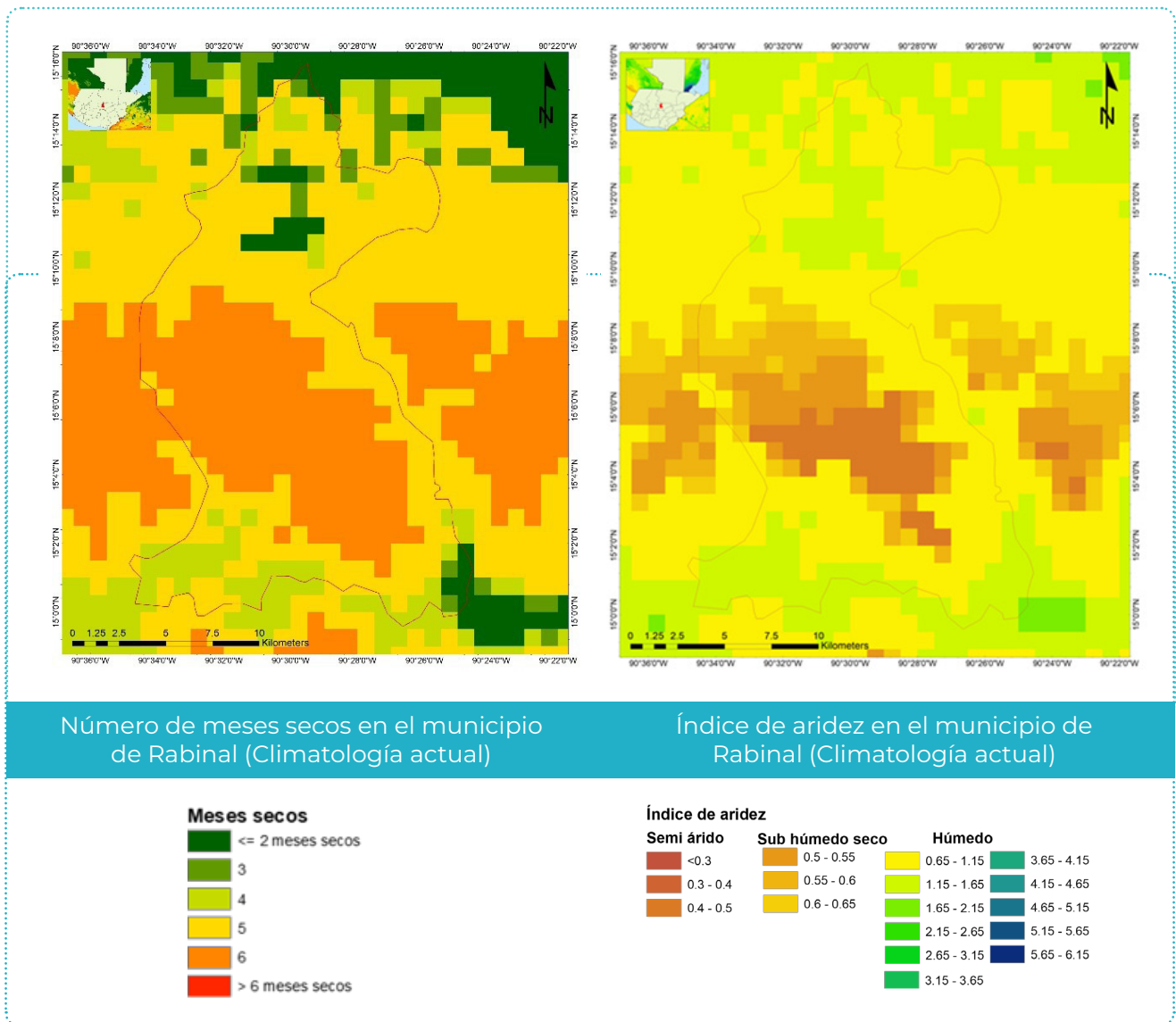
Figura 24. Número de meses secos, índice de aridez y evapotranspiración potencia en el municipio del Rabinal, Baja Verapaz, Guatemala, según climatología 1960-1990
