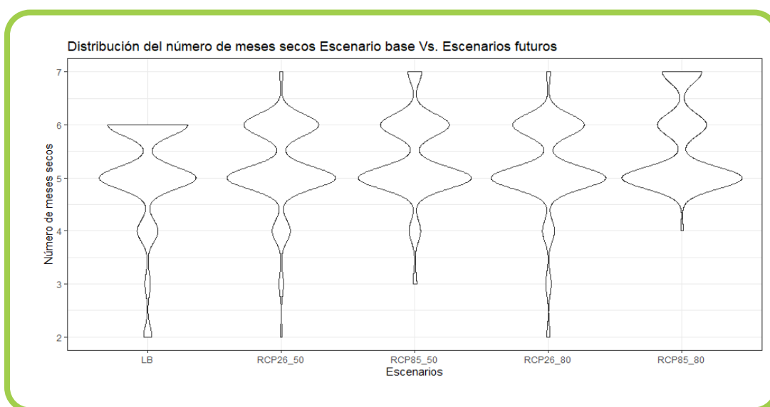
Figura 26. Comparación en la distribución de meses secos entre la línea base y los escenarios futuros para Rabinal, Baja Verapaz, Guatemala
