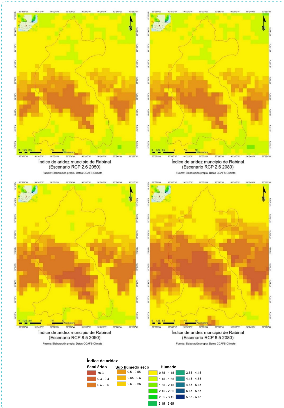
Figura 27. Cambios en el índice de aridez, entre la línea base y los escenarios futuros para Rabinal, Baja Verapaz, Guatemala
